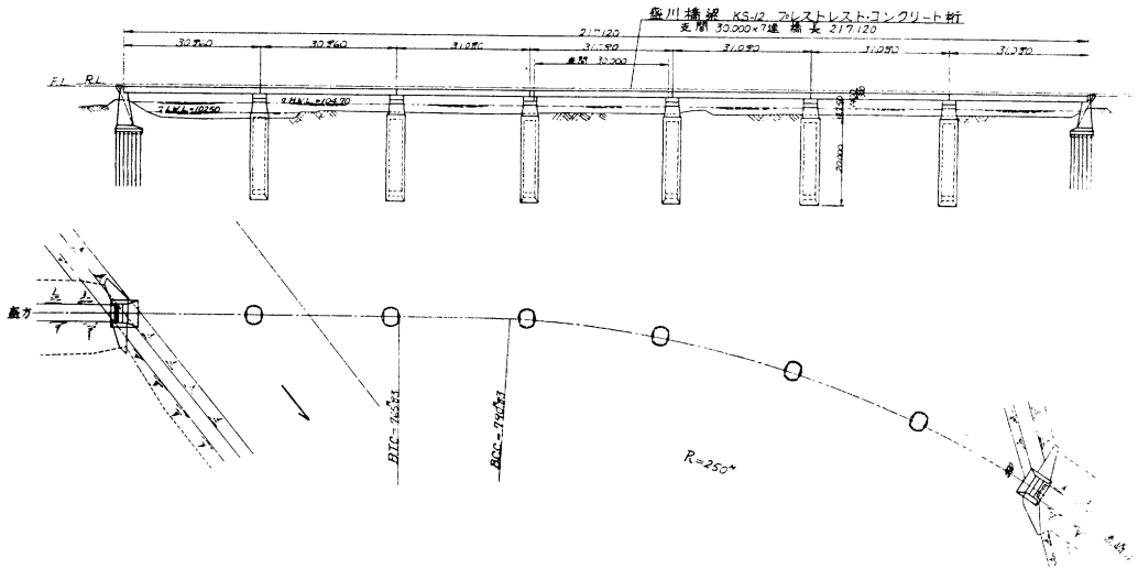
図一1 盛川橋梁一般図
