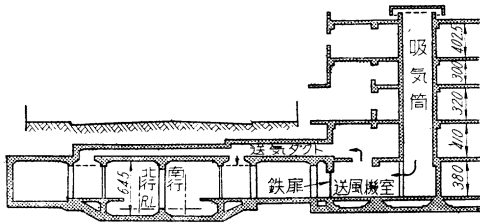
図三 岸里停留場吸気筒部
