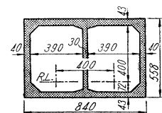
図四 函型トンネル断面
