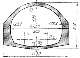
図五 拱型トンネル断面
