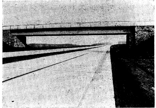
写真一3 エルデ橋(ドイツ)1938 年建設
