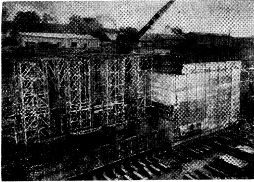
写真一2 プレスト港の PC によるケーソン工事
