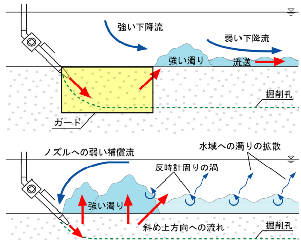
図-5 濁りの拡散メカニズム（上：CASE-A 下：CASE-B）
