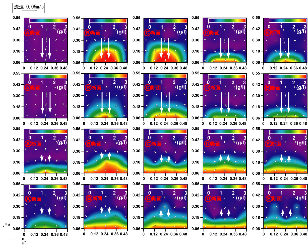
図-10 濁度分布および流速ベクトル（横断方向）（左から x^*=0, 0.36, 0.48, 0.73, 0.97 断面） （1行目：CASE-Aの結果Ⅰ 2行目：CASE-Aの結果Ⅱ 3行目：CASE-Bの結果Ⅰ 4行目：CASE-Bの結果Ⅱ）
