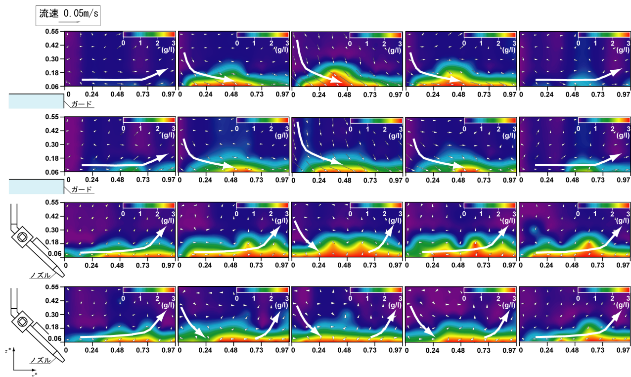
図-9 濁度分布および流速ベクトル（縦断方向）（左から y^*=0, 0.12, 0.24, 0.36, 0.48 断面） （1行目：CASE-Aの結果Ⅰ 2行目：CASE-Aの結果Ⅱ 3行目：CASE-Bの結果Ⅰ 4行目：CASE-Bの結果Ⅱ）
