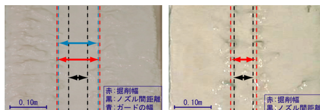
図-8 掘削幅（左：CASE-A 右：CASE-B）
