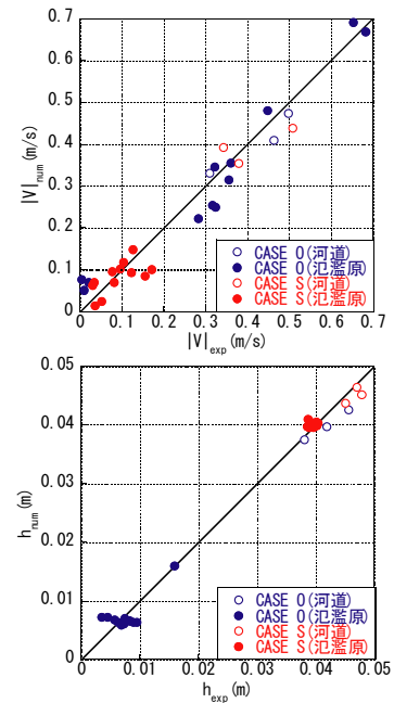
図-10 流速と水深の比較 (上:流速 下:水深)
