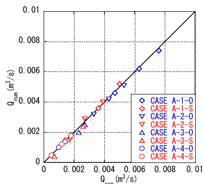
図-11 破堤氾濫流量の比較(本解析法)
