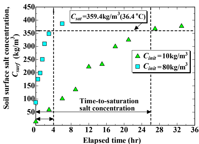
図-4 土壌表面塩濃度 C_{surf} の経時変化
