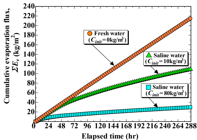
図-5 積算蒸発量 \Sigma E_v の経時変化
