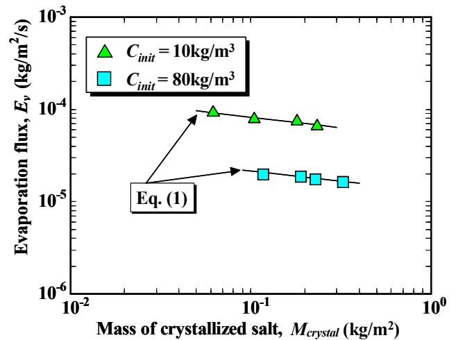
図-8 析出塩量 M_{crystal} と蒸発フラックス E_v の関係
