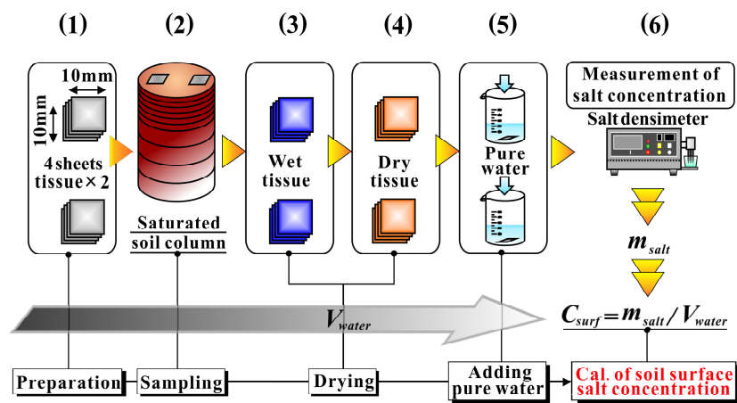
図-3 吸水紙法
