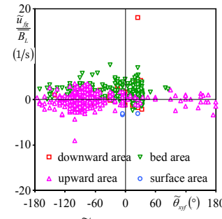
図-13(d) 瞬間魚向 \tilde{\theta}_{xyf} と瞬間対地速度 \tilde{u}_{fg} の関係
