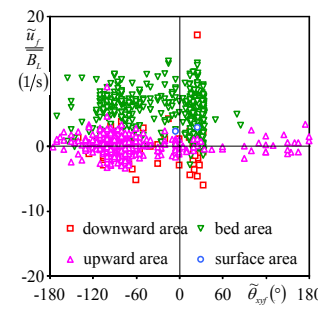
図-13(c) 瞬間魚向 \tilde{\theta}_{xyf} と瞬間遊泳速度 \tilde{u}_f の関係
