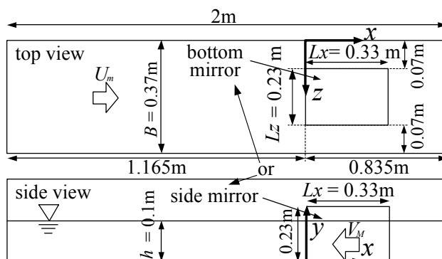
図-1 実験装置
