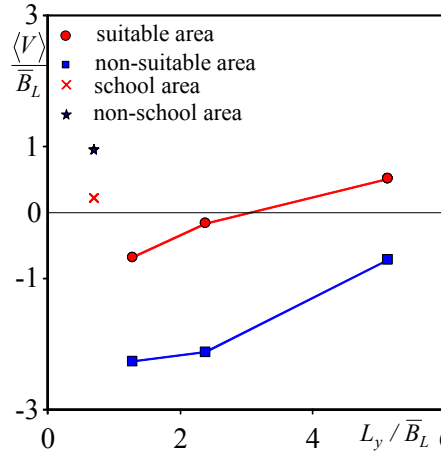
図-8(b) 休憩・非休憩場所の鉛直方向流速と段落ち高さの関係
