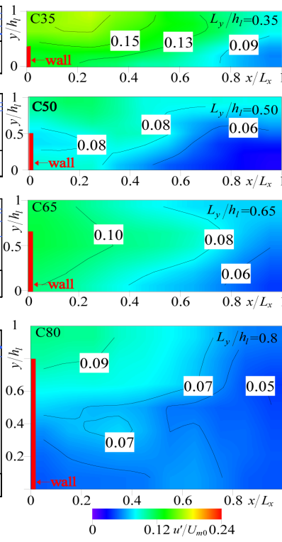
図-3(a) 乱れ強度 u'/U_{m0}
