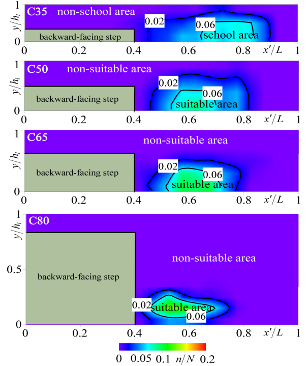
図-4 存在率コンター
