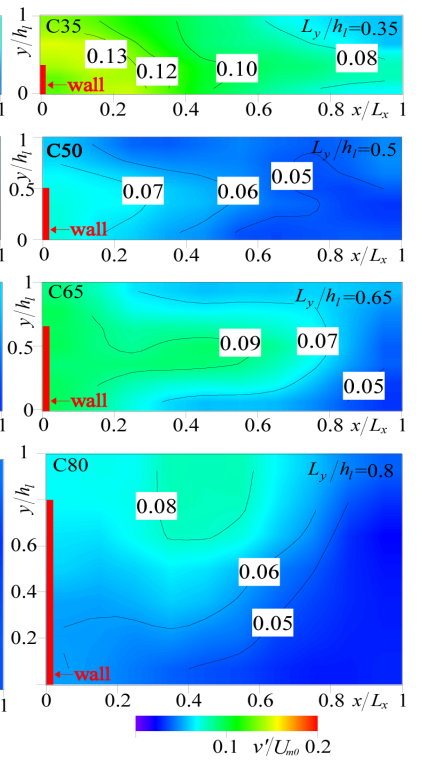
図-3(b) 乱れ強度 v'/U_{m0}
