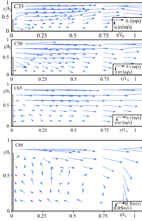
図-2 流速ベクトル
