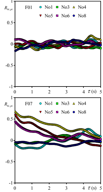
図-11 水深と圧力の相互相関係数
