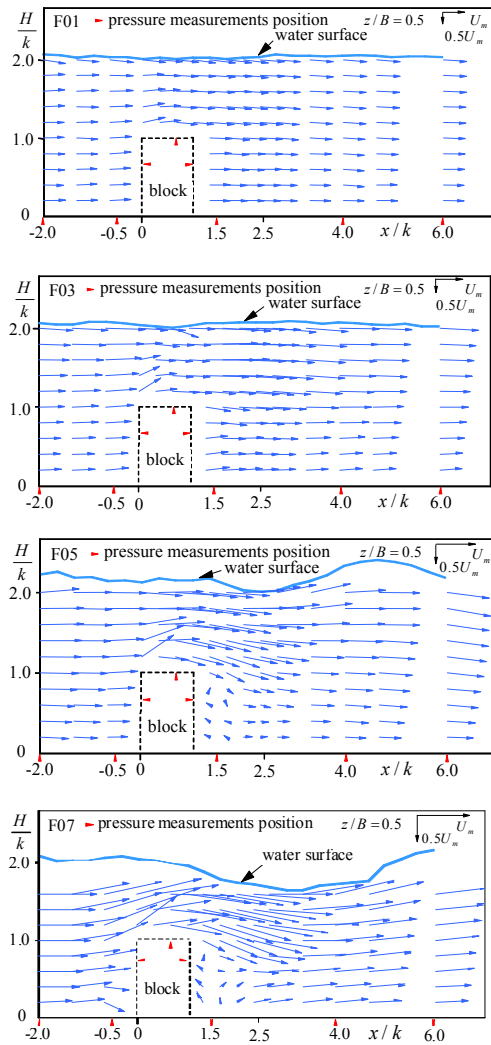
図-3 流速ベクトル図
