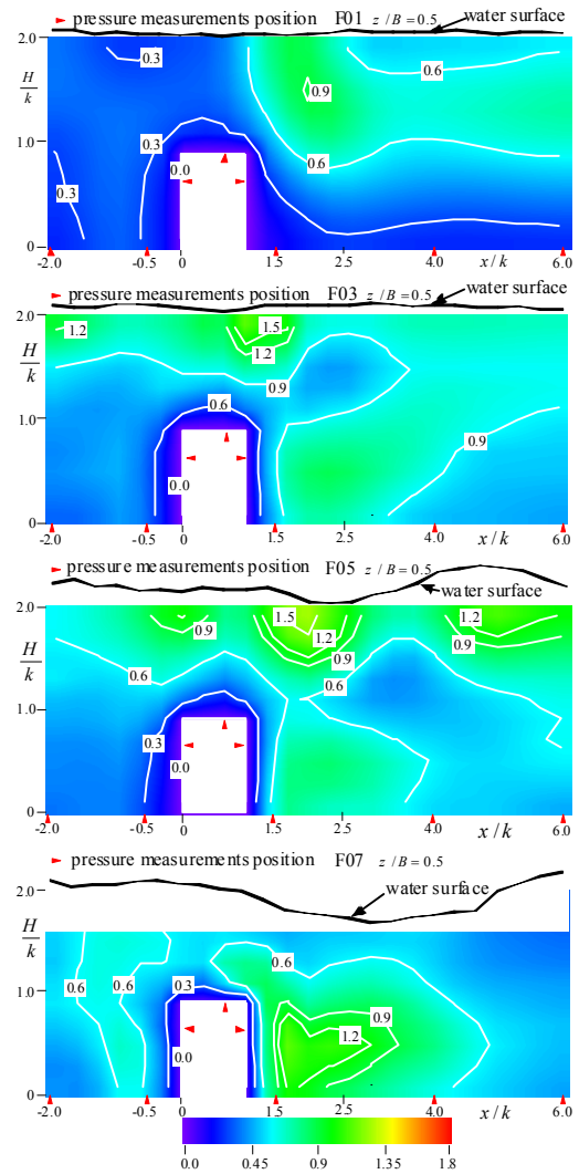
図-4 v'/u' のコンター図
