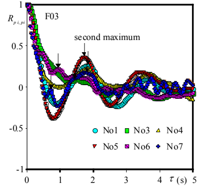
図-7(a) 圧力の自己相関係数
