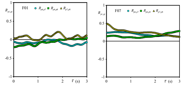
図-12 No. 6, No. 7およびNo. 8の圧力の相互相関係数
