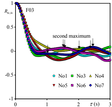
図-7(b) 水深の自己相関係数
