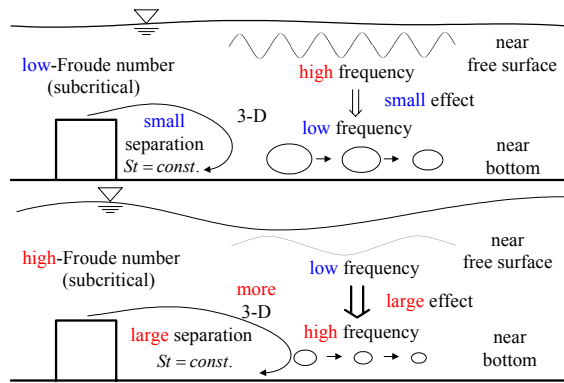
図-13 矩形ブロック背後の流れ場の模式図
