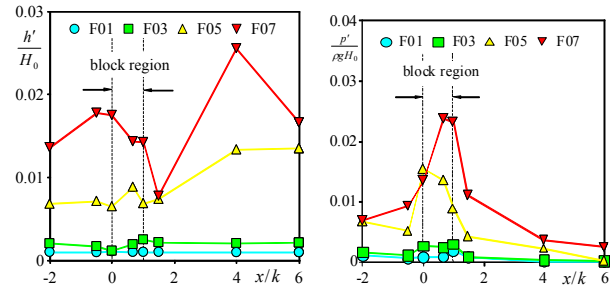
図-5 水深のRMS値
