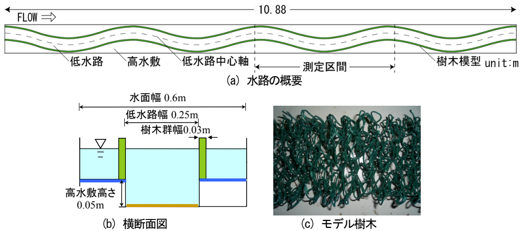
図-1 実験装置
