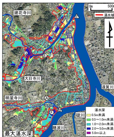
図-8 湛水域の比較
