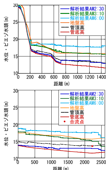
図-7 下水道幹線網の水位・ピエゾ水頭の経時変化 (上：西1号幹線，下：西部幹線)
