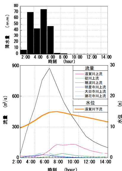
図-5 解析に用いたハイドログラフと流量・水位ハイドログラフ
