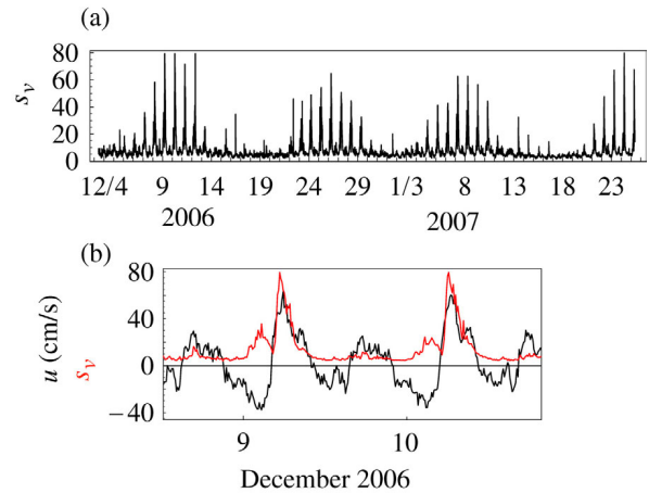
図-8 体積後方散乱係数(懸濁粒子濃度)の経時変化
