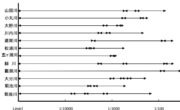
図-7 12 河川の魚類相区分と河床勾配
