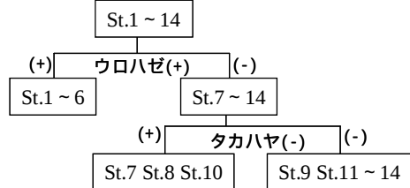
図-4(a) 球磨川における TWINSpan 分析結果
