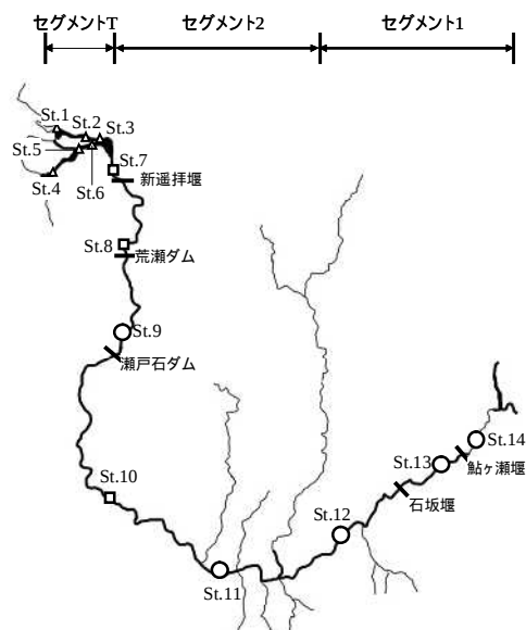
図-4(b) 球磨川におけるセグメントと魚類相区分
