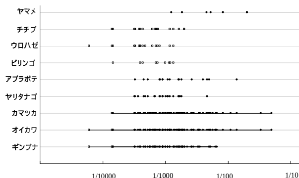
図-6 代表的な種の出現地点の河床勾配
