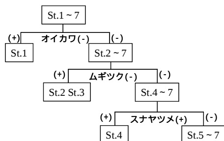
図-3(a) 大分川における TWINSpan 分析結果
