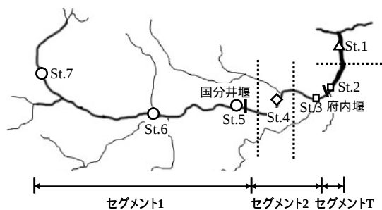
図-3(b) 大分川におけるセグメントと魚類相区分
