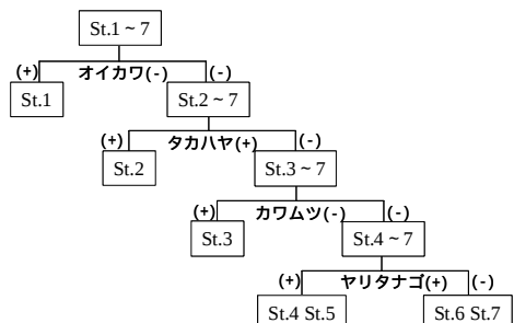
図-2(a) 筑後川における TWINSpan 分析結果
