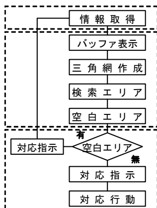
図-7 情報収集支援システムのワークフロー
