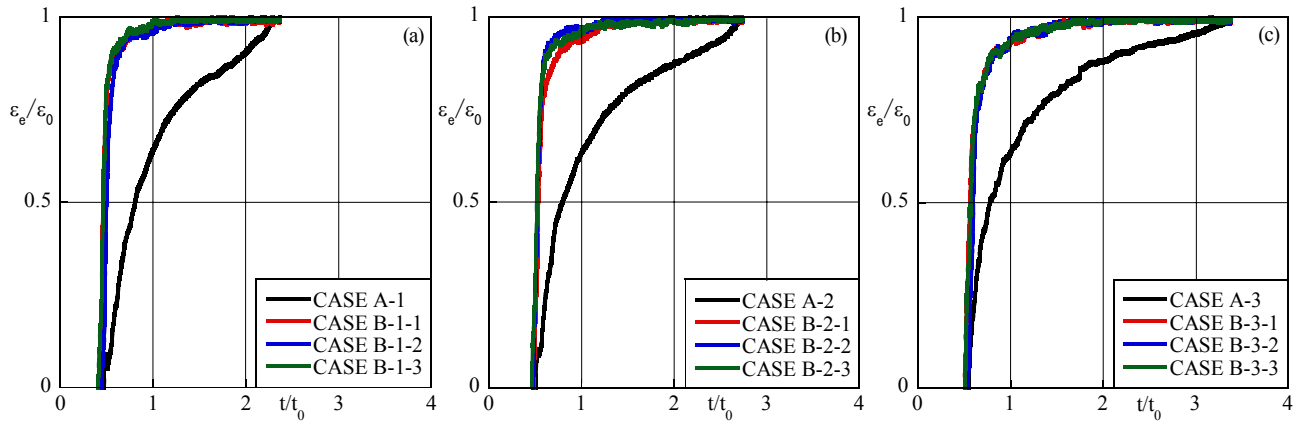
図-3 越流水の相対密度差の時系列 ((a) F_0=0.70 , (b) F_0=0.86 , (c) F_0=1.08 )
