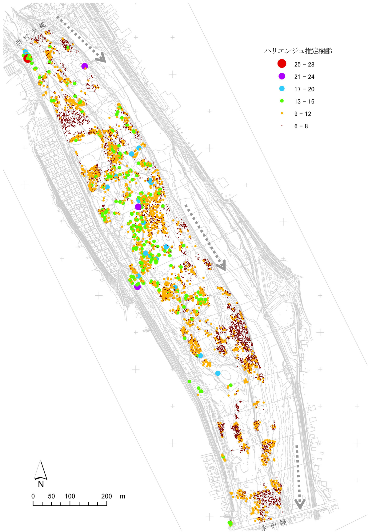
図-3 毎木調査によるハリエンジュ生育位置図と推定樹齢 21) (矢印は滞筋における流下方向を示す。調査対象地は永田橋から羽村大橋までの高水敷右岸である。)
