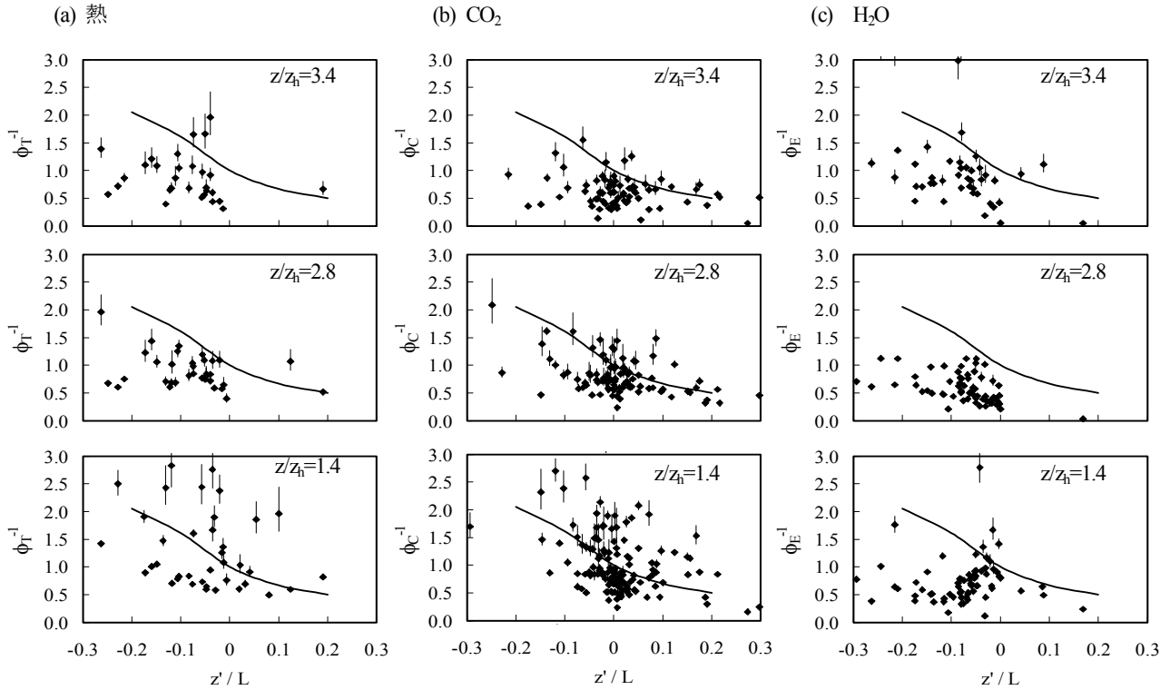
図-2 異なる高度における(a)熱, (b)CO 2 , (c)H 2 O の無次元拡散係数と大気安定度. 高度は平均建物高さで無次元化し, それぞれのグラフに示した. 実線は既存の無次元拡散係数 (Dyer and Hicks, 1970 8) , Businger et al., 1971 9) ) を示す.
