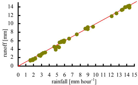
図-10 流出量と降雨強度の関係（7時間移動平均値）
