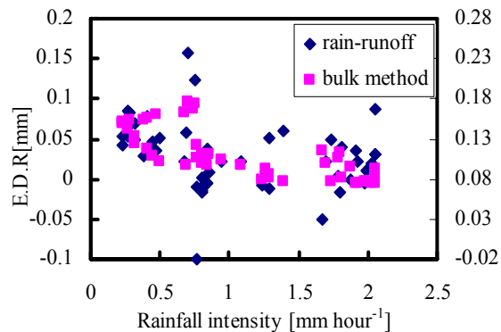
図-12 降雨中蒸発量の降雨強度依存性（7時間移動平均値） 右軸：バルク法によるEDR 左軸：残差によるEDR
