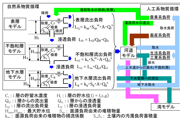
図-3 流域物質循環モデルの構造
