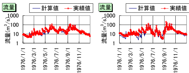
図-7 河川流量の実測値と計算値(荒川・1976年)
