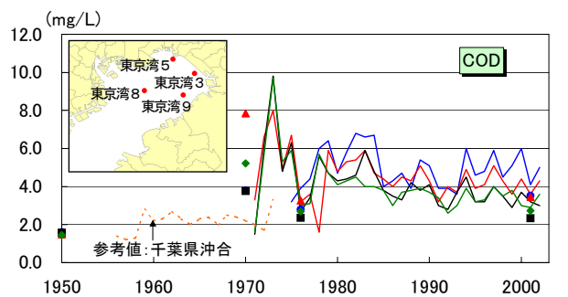
図-10 東京湾の実測水質の変遷と計算結果との比較(COD)
