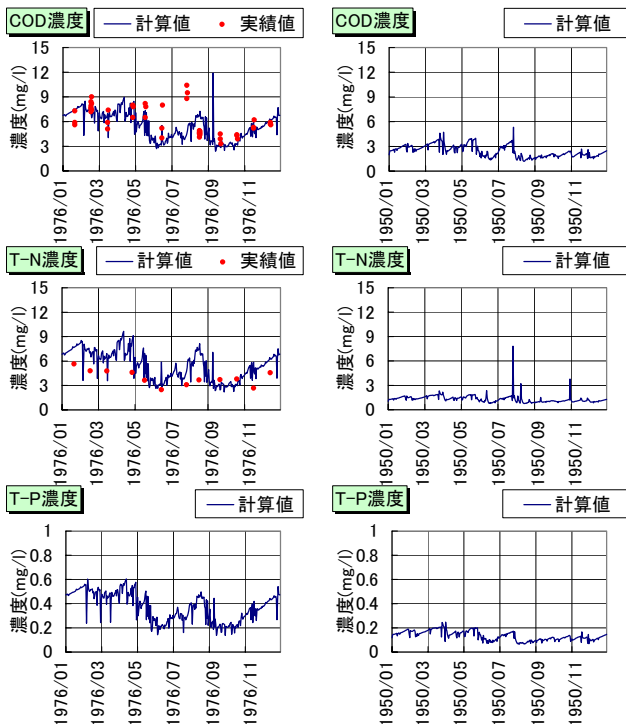
図-8 河川水質の実測値と計算値(荒川・笹目橋地点)
