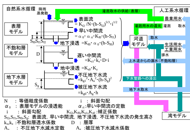
図-2 流域水循環モデルの構造
