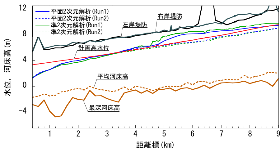
図-6 計画高水流量時の水位の解析結果
