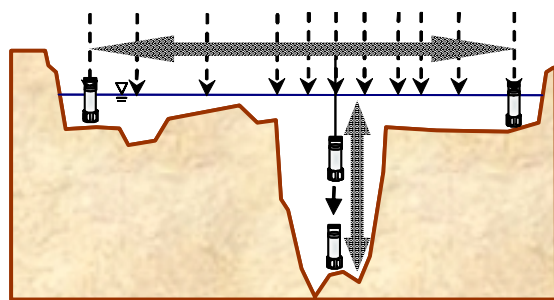
図-1 濁度計付きCTDセンサーの使用方法
