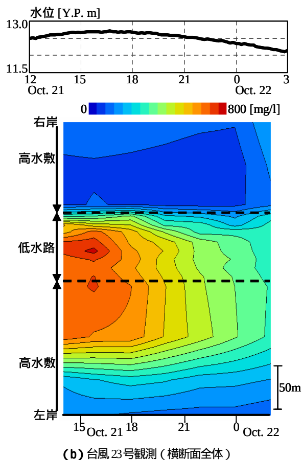
図 - 6 水深平均 SS の横断分布に関する時間変化 (新関宿橋)
