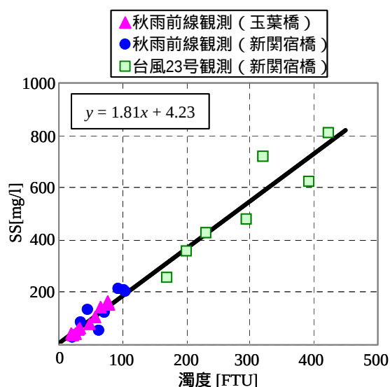
図-2 濁度とSSのキャリブレーション結果
