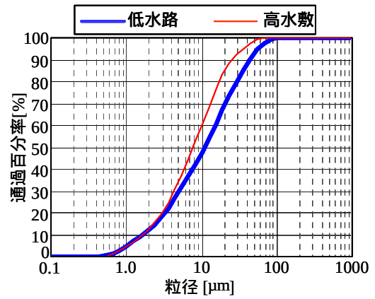
図 - 4 浮遊土砂の粒径分布 (台風23号観測, 新関宿橋)
