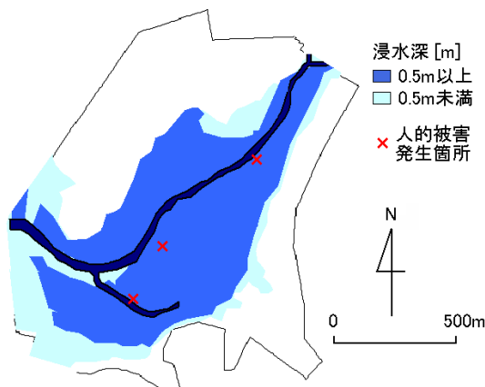
図-3 中島川周辺の浸水実績 7)
