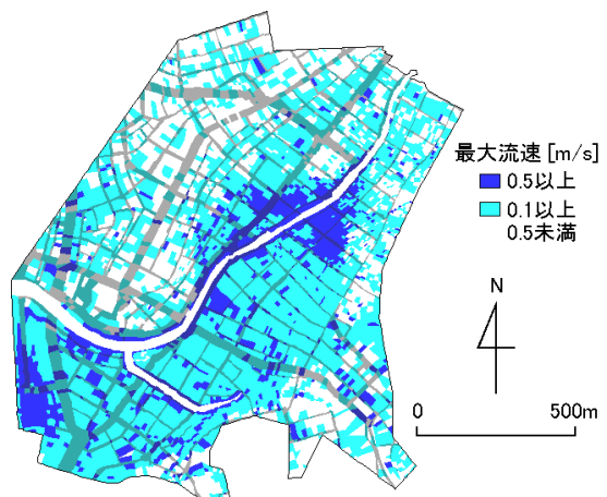
図-10 最大流速
