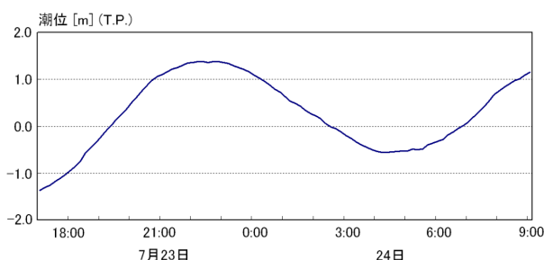
図-8 実測河口潮位 11)
