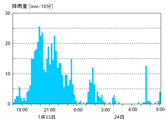
図-2 長崎海洋気象台の10分間雨量
