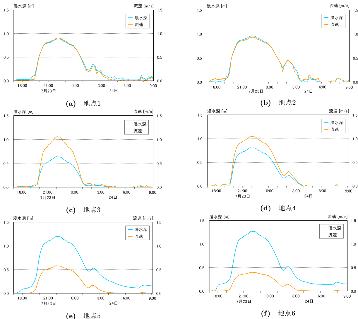
図-13 領域内各地点の浸水深・流速の時間的変化
