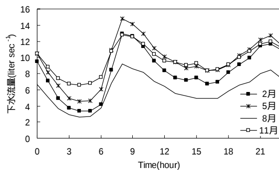
図-3 季節別の下水流量の時間変動
