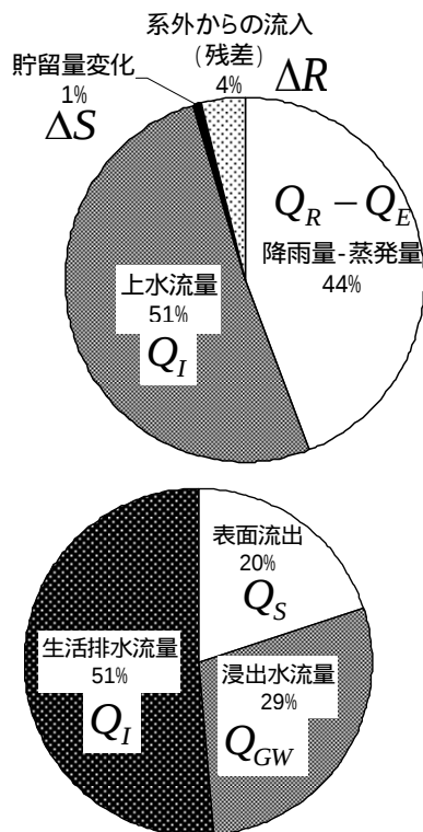
図-9 (上) 系内に供給される水の内訳 (下) 系外に流出する水量の内訳
