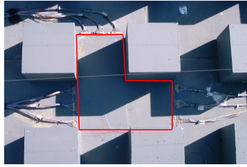
図-2 熱流板の設置(床面、赤線の枠内)
