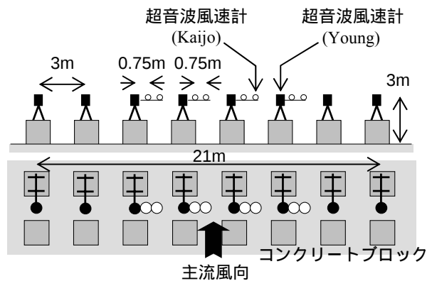
図-5 超音波風速計配置図(水平分布)
