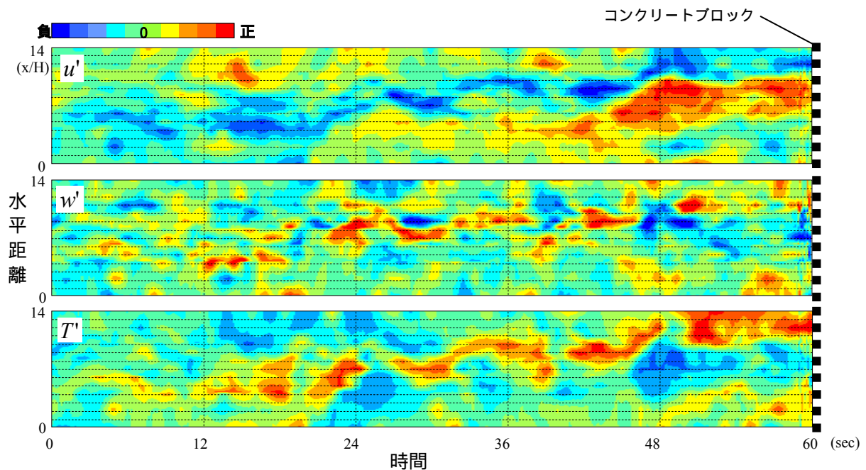
図-13 各種時間変動量の水平-時系列分布 (2005年8月4日16時32分より1分間) 平均風速: 2.2 \text{ m s}^{-1} , 高度: 2H , コンター範囲: u' : -2 \sim 2 \text{ m s}^{-1} , w' : -1 \sim 1 \text{ m s}^{-1} , T' : -2 \sim 2 \text{ K}
