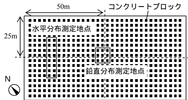
図-3 屋外都市モデル略図
