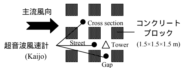
図-4 超音波風速計配置図(鉛直分布)
