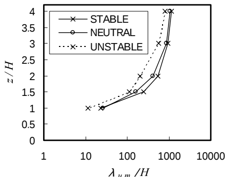
図-12 スペクトル解析による卓越波長の高度変化
