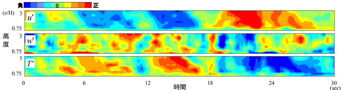
図-8 各種時間変動量の鉛直-時系列分布
