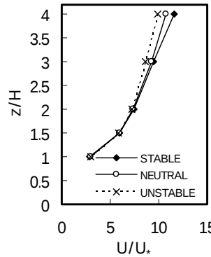
図-6 平均風速鉛直分布
