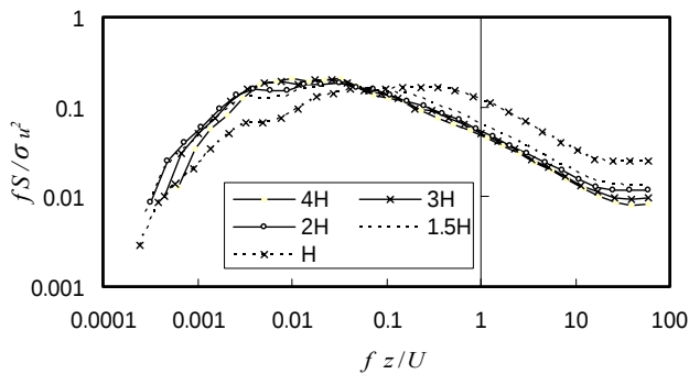
図-11 水平主流風速の周波数解析（不安定時）
