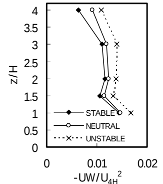
図-7 運動量鉛直分布
