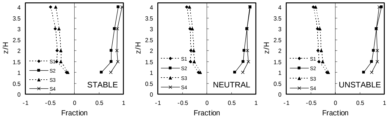
図-10 安定度別四象限解析の鉛直分布 (左: 安定、中: 中立、右: 不安定)
