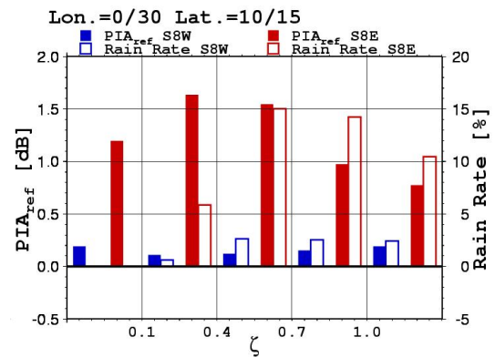
図-10 サヘル(0-30E, 10-15N)におけるPIA ref および降雨強度。S8WとS8Eの場合のORGに対する変化で表示。
