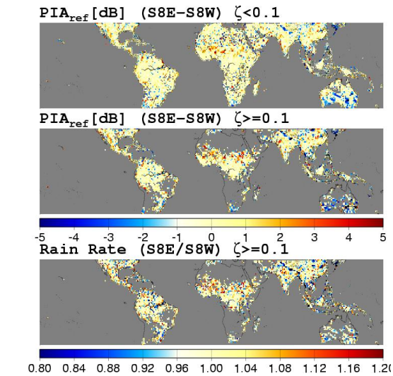
図-9 S8WをS8Eに変えた場合の変化。(上) \zeta < 0.1 の場合のPIA ref の増加。(中) \zeta \geq 0.1 の場合のPIA ref の増加。(下)降雨強度の増加率。
