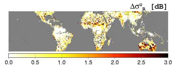
図-5 \zeta < 0.1 の場合の \Delta \sigma_R のグリッドごとの平均値。 \Delta \sigma_R > 0 の場合のみ表示。
