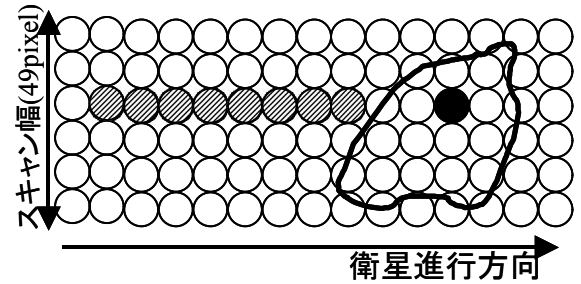
図-2 空間参照法の説明。太線内を降雨域とする。黒塗り示した対象ピクセルに空間参照法を適用する場合、ハッチをかけた8つのピクセルを利用する。
