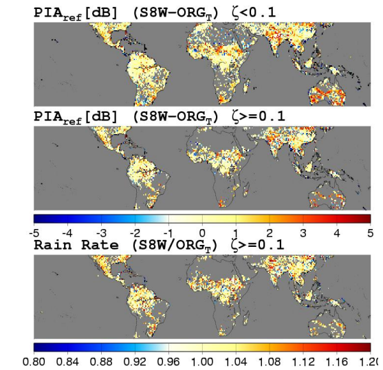
図-6 ORGの時間参照法をS8W(空間参照法)に変えた場合の変化。(上) \zeta < 0.1 の場合の PIA_{ref} の増加。(中) \zeta \geq 0.1 の場合の PIA_{ref} の増加。(下)降雨強度の増加率。
