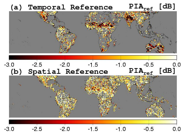
図-3 \zeta < 0.1 の場合の PIA_{ref} のグリッドごとの平均値。 PIA_{ref} が負の場合のみ表示。(a)は時間参照法、(b)は空間参照法の場合。
