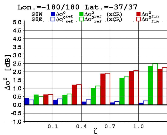
図-12 \Delta\sigma_{ref}^0 、非一様性の補正を考慮して計算した \Delta\sigma_{ref}^0 、 \Delta\sigma_{fin}^0 の比較。S8WおよびS8Eの陸上全体について平均値。
