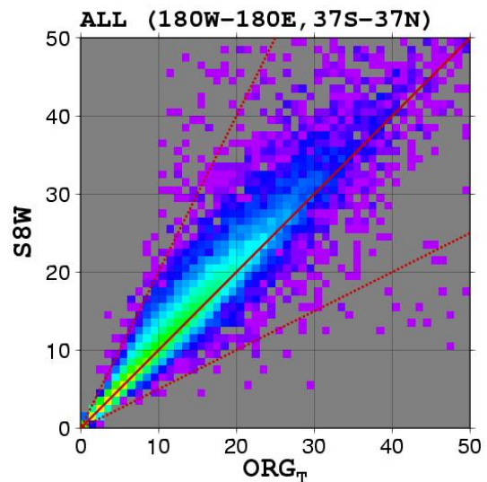
図-8 ORGの時間参照法とS8W(空間参照法)による降雨強度[mm/h]の比較。2次元ヒストグラムで表示。暖色系は高い頻度を示す。
