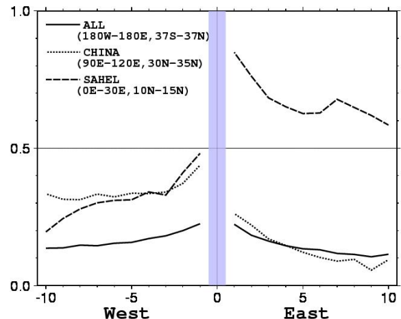
図-4 降雨域からの距離別の \Delta \sigma_m 平均値。
