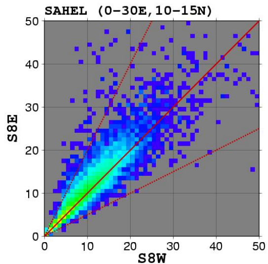
図-11 S8WとS8Eによる降雨強度[mm/h]の比較。2次元ヒストグラムで表示。
