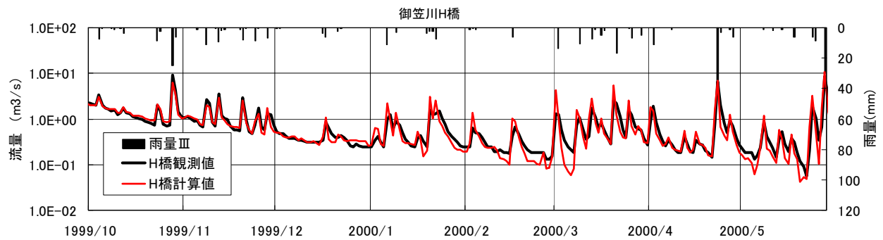
図-6 流出-涵養モデルの検証結果
