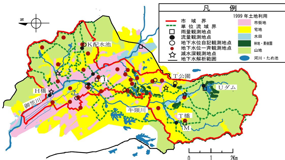
図-2 主な調査・観測位置及び土地利用状況
