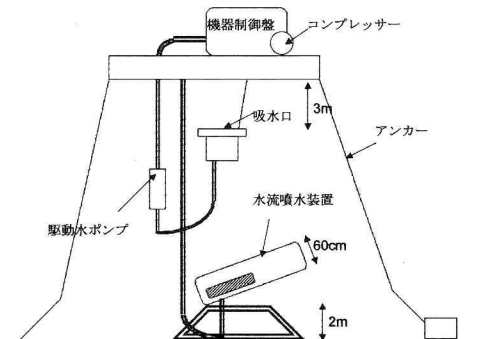
図-6 水流発生装置
