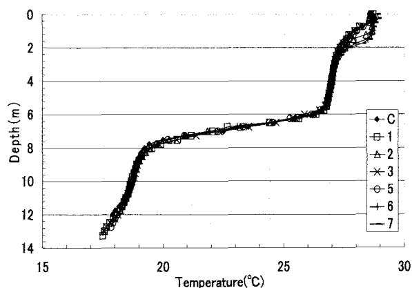
図-9 水温分布(8/25)
