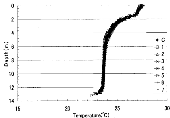
図-10 水温分布(9/14)
