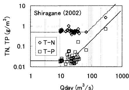
図-7 矢作川中流 (古単地区, 44.0 km 地点) における日平均流量 Q_{\text{day}} と全窒素濃度 TN , 全リン濃度 TP の関係
