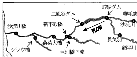
図-8 沙流川における洪水時の観測地点
