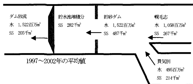
図-11 年間の水収支及びSS収支 (1997-2002の平均)
