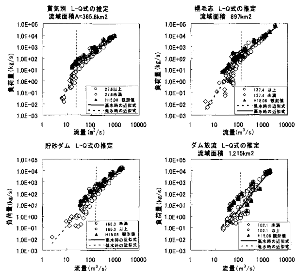
図-9 二風谷ダム貯水池前後における負荷量式
