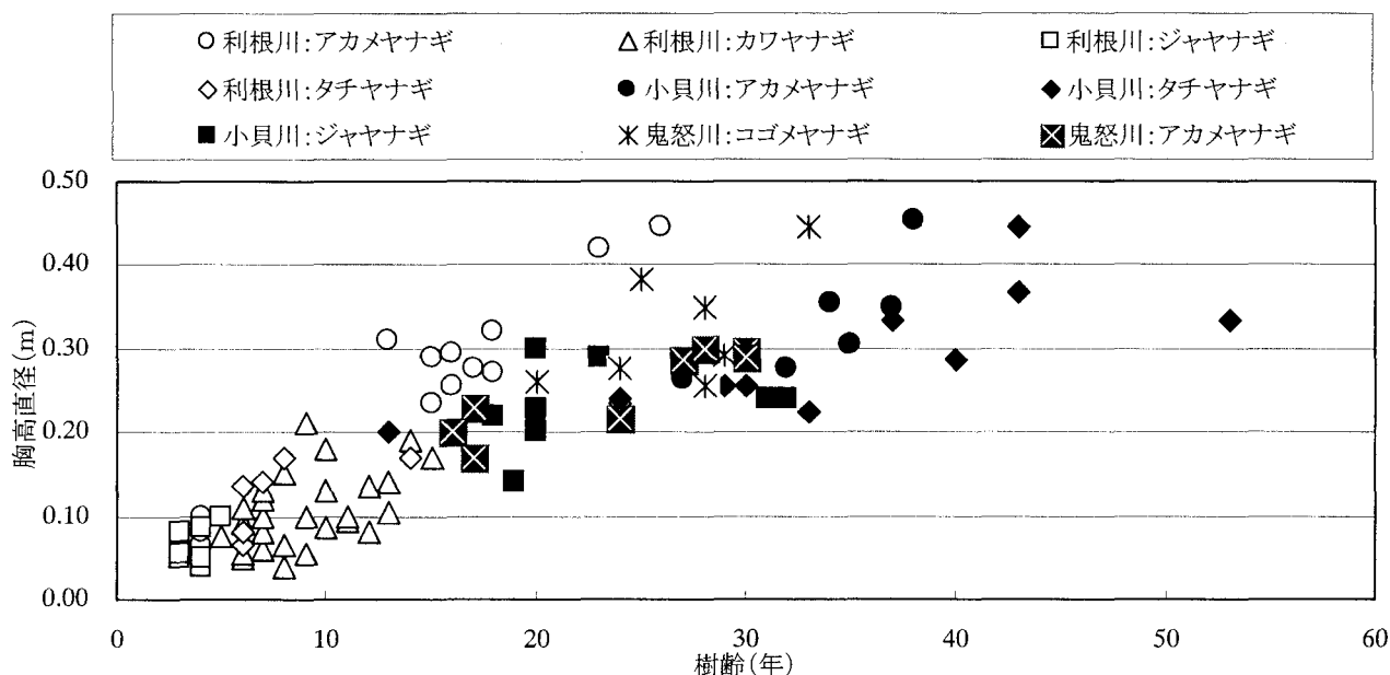
図-7 小貝川、利根川、鬼怒川の樹齢と胸高直径との関係
