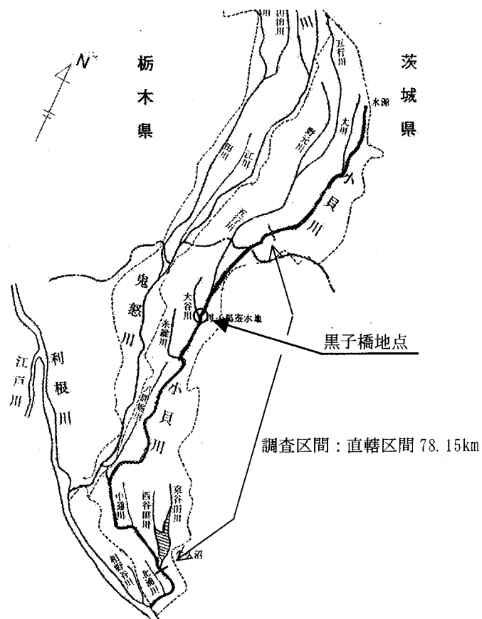
図-1 小貝川流域平面図 S=1:900000
