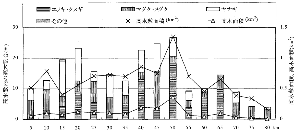
図-6 高木別の高水敷面積に対する高木面積の割合（小貝川）
