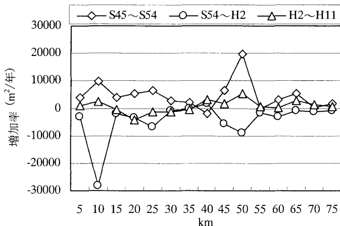
図-4 高木群増加率(5km ピッチ)
