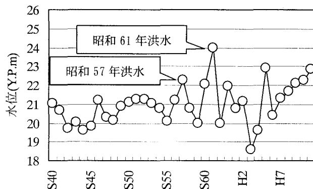
図-3 小貝川黒子地点での年最高水位
