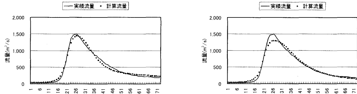
図-7 流域モデル+河道モデルによる全流出量の再現結果 (左：2段タンク型，右：1段タンク型) (上渚滑地点 1998.9.16 1:00-9.18 24:00)
