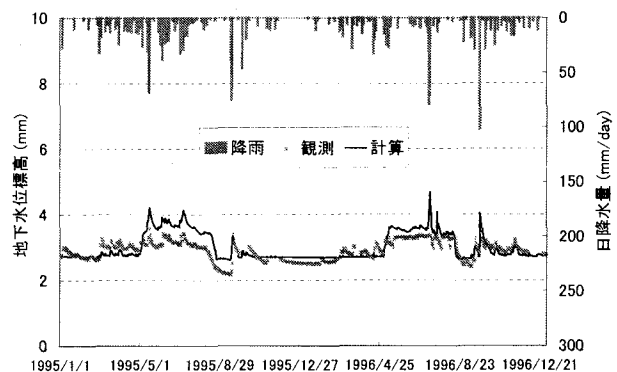
図-5 地下水位の比較（前原川市場）
