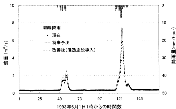
図-11 浸透施設有無による河川流量の比較 (八栄橋地点)
