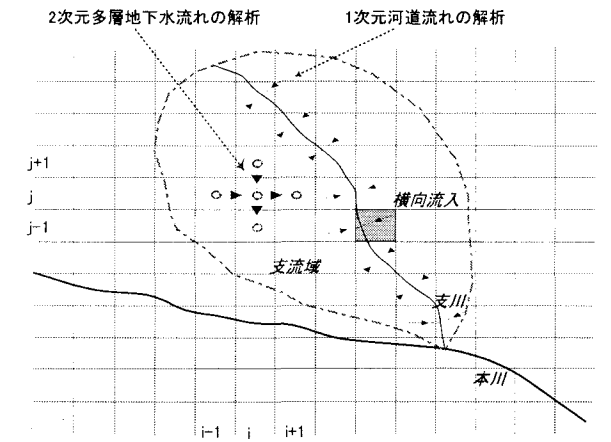
図-2 モデルの平面構造
