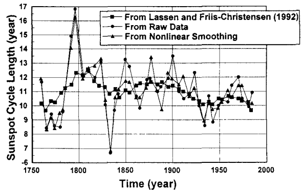
図-4 太陽黒点周期長
