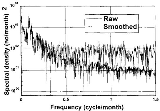
図-2 太陽黒点時系列のパワースペクトル
