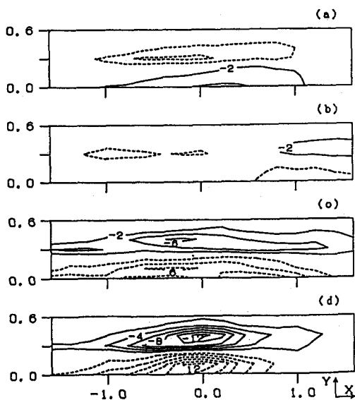
図8 各X Y断面内の渦度 \omega_z の
