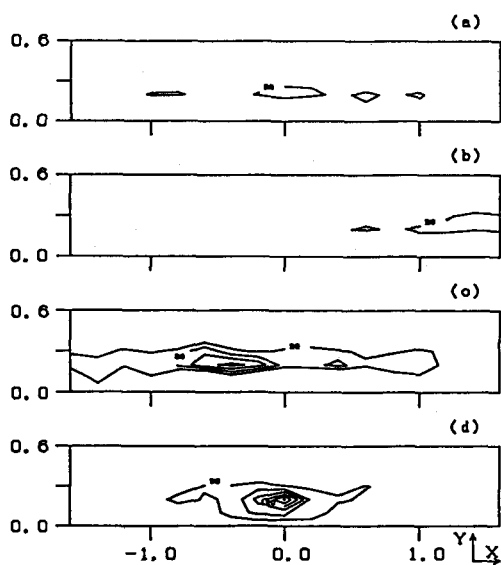
図11 各X Y断面内の平均レイノルズ応力
