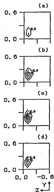
図7 各Y Z断面内の渦度 \omega_x の
