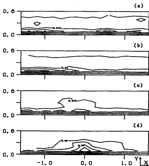
図10 各X Y断面内の乱れのr. m. s.
