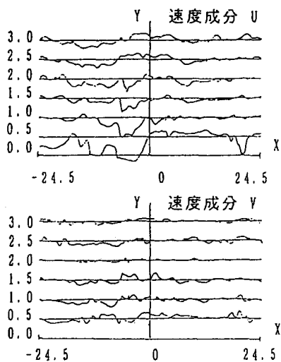
図12 速度変動のなま波形 (位相90~100度)
