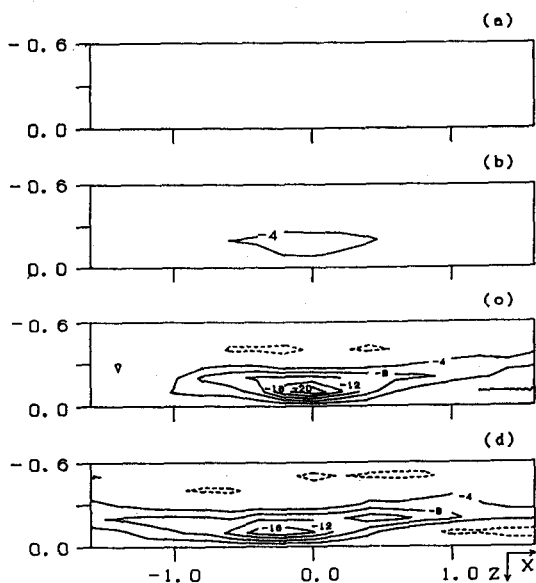
図6 各X Z断面内の渦度 \omega_y の
