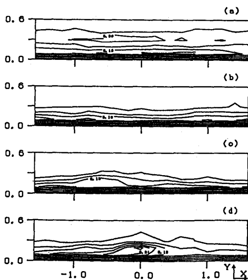
図9 各X Y断面内の乱れのr.m.s.
