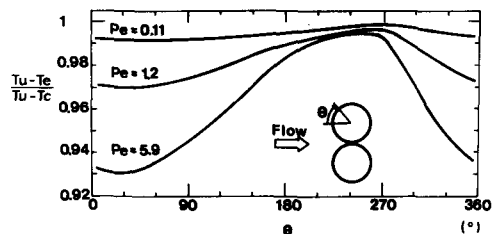
図-9 HP外壁周方向温度分布
