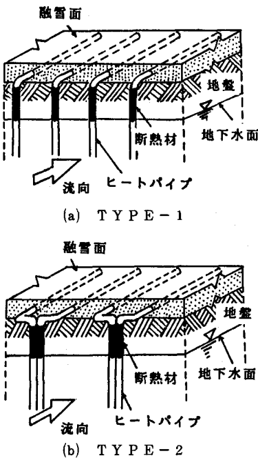
図-1 HP融雪装置
