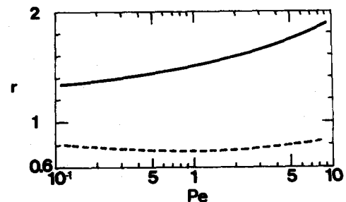
図-13 HPへ流入する熱量の比較
