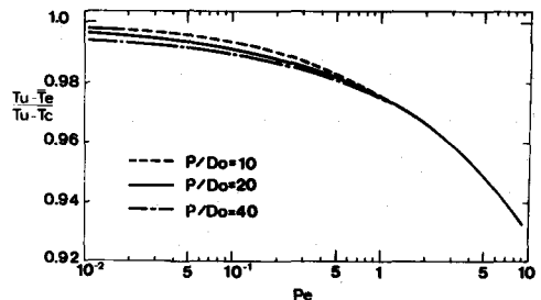
図-5 HP外壁平均温度
