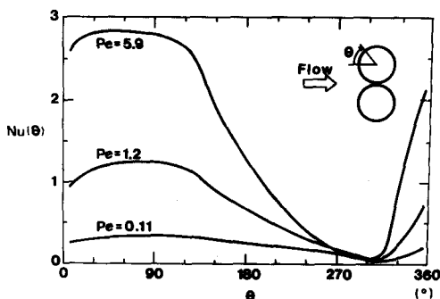
図-11 HP外壁局所ヌセルト数分布
