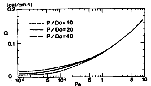
図-8 HPへ流入する熱量
