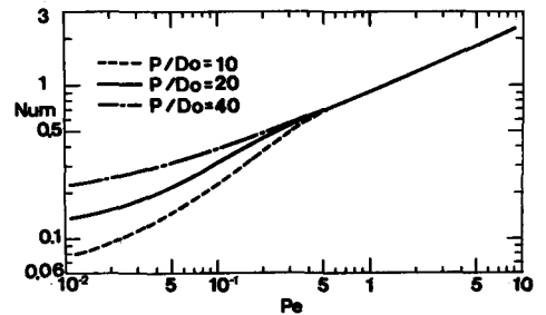
図-7 HP外壁平均ヌセルト数
