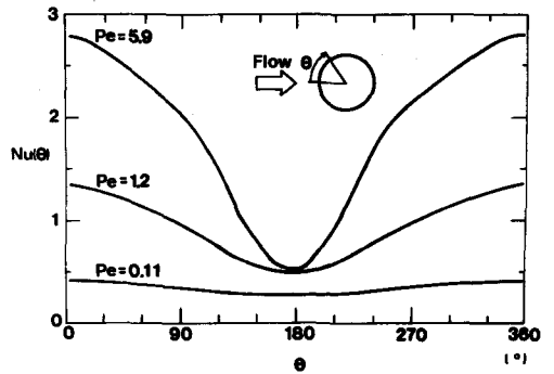
図-6 HP外壁局所ヌセルト数分布
