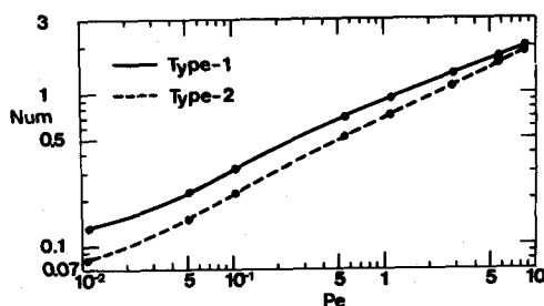
図-12 HP外壁平均ヌセルト数
