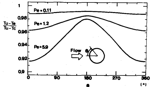
図-4 HP外壁温度分布
