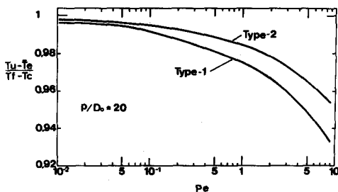
図-10 HP外壁平均温度
