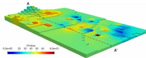
図-13 神戸市灘区の3次元地盤グリッドモデル（伊藤ら，2022の図-3）
