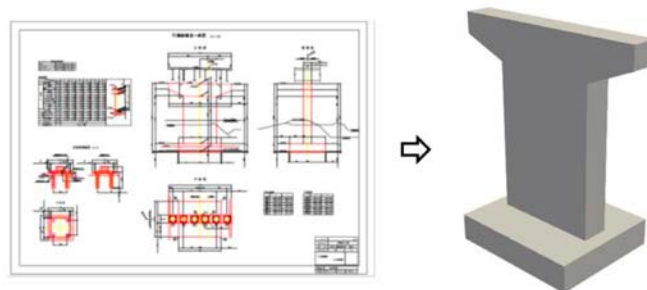
図-6 2次元CADデータから3次元モデルを生成
