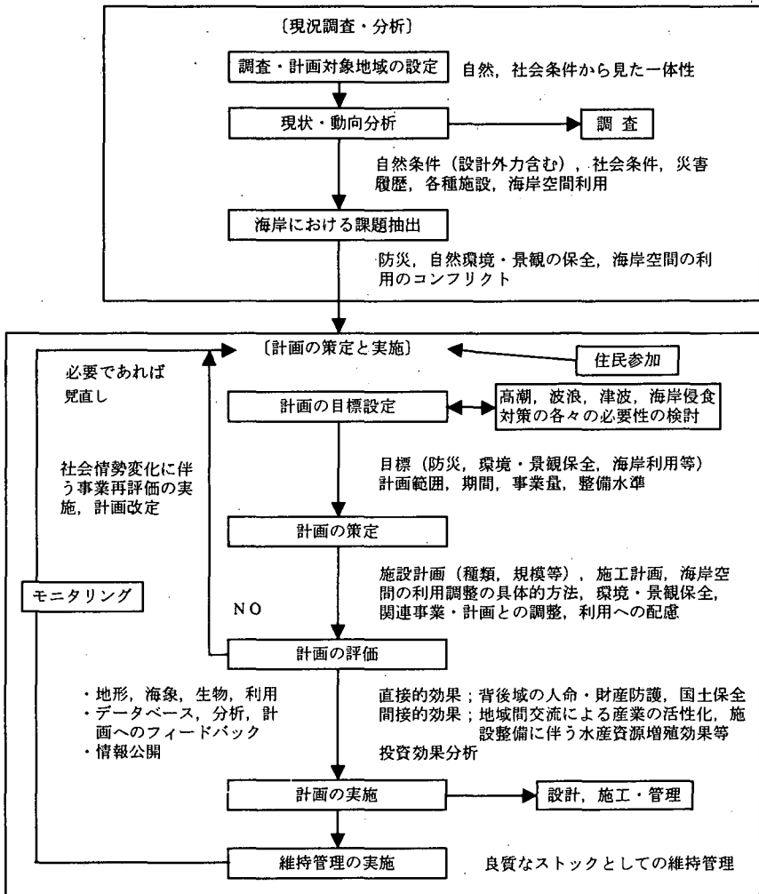
図-2 海岸施設設備計画策定の流れ
