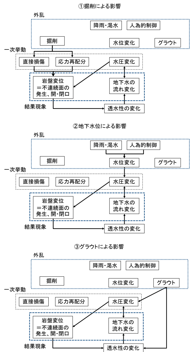
図-3 様々な外乱による応力-水連成挙動の概念
