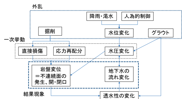
図-2 応力-水連成挙動における相関
