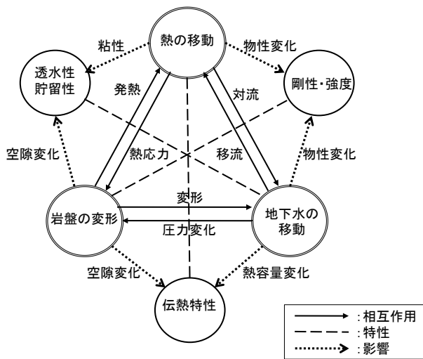
図-1 岩盤における応力-熱-水連成挙動の概念
