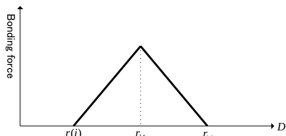
図-4 ボンディング力
