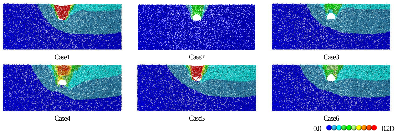
図-5 変位分布図（変位収束後）
