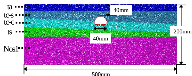
図-1 多層地盤モデル (H=1.0D)
