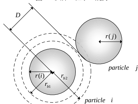
図-3 ボンディング力の作用領域
