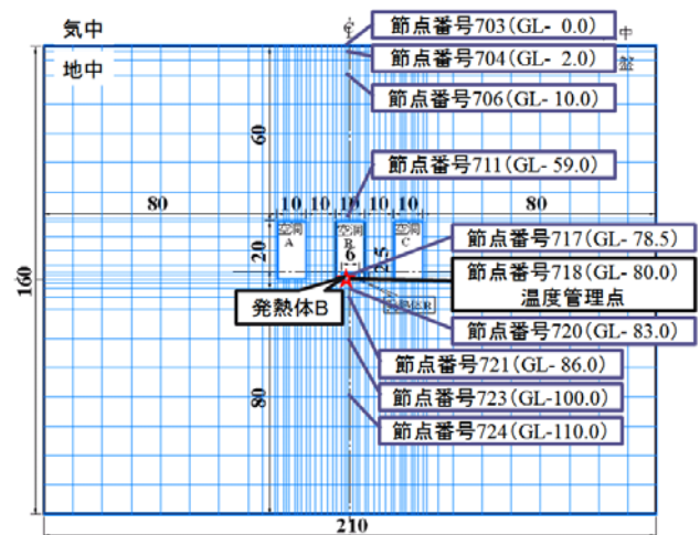
図-3 解析モデル
