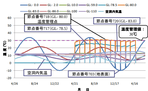
図-10 空洞内気温内に設置した発熱体を冷却した場合の発熱体と地盤内部の温度変化(管理目標値:30℃)
