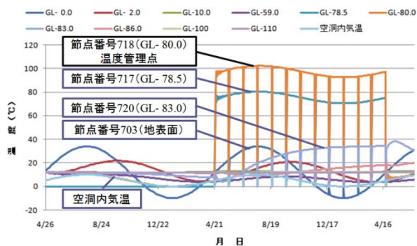
図-9 発熱体を冷却しないで空洞内部に放置した場合の発熱体と地盤内部の温度変化(空洞外気温による熱伝達)
