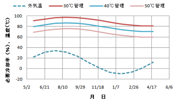
図-8 温度管理値と必要冷却率の変化(外気温による熱伝達の場合)
