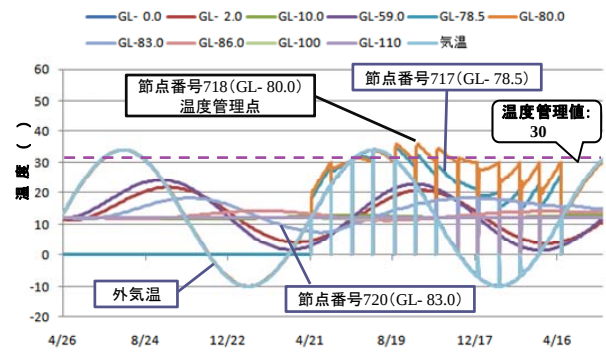
図-6 外気温内に設置した発熱体を冷却した場合の発熱体と地盤内部の温度変化(管理目標値:30℃)
