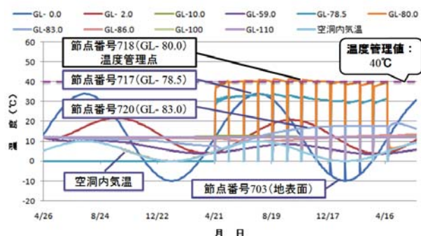
図-11 空洞内気温内に設置した発熱体を冷却した場合の発熱体と地盤内部の温度変化(管理目標値:40℃)
