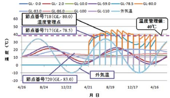
図-7 外気温内に設置した発熱体を冷却した場合の発熱体と地盤内部の温度変化(管理目標値:40℃)
