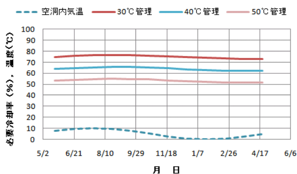
図-12 温度管理値と必要冷却率の変化(空洞内気温による熱伝達の場合)
