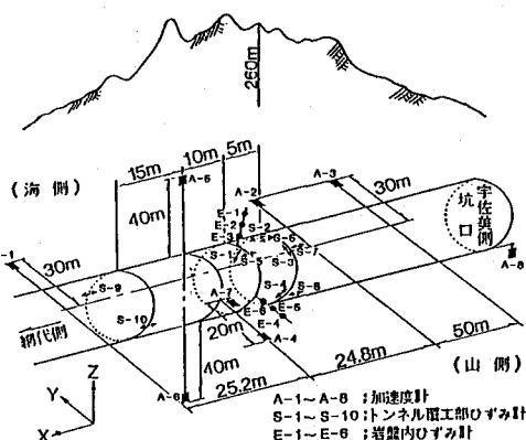
図-1 地震観測計器配置図
