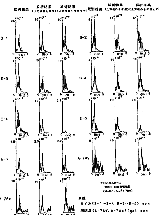
図-8 過渡応答解析結果と観測値の比較 (フーリエスペクトル)
