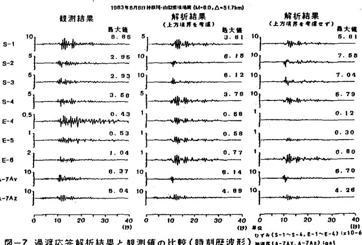
図-7 過渡応答解析結果と観測値の比較 (時刻歴波形) 加振波 (A-7Ay, A-7Az) 1 \text{ gal}
