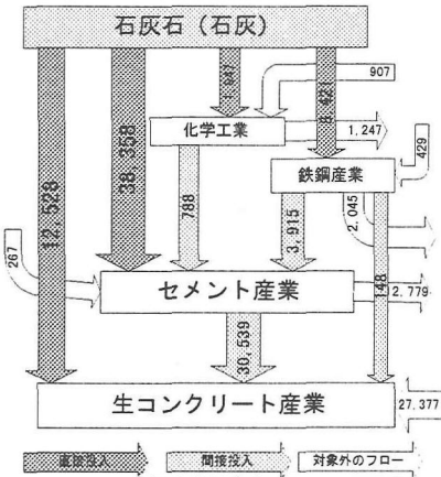
図2 石灰石の収支フロー (単位：千 t (Ca換算値))
