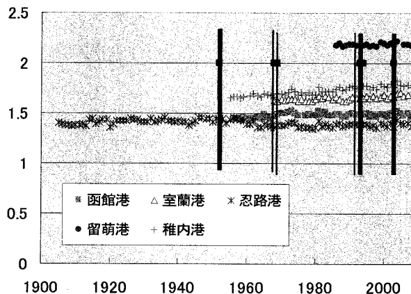
図-5 年平均潮位（西側）
