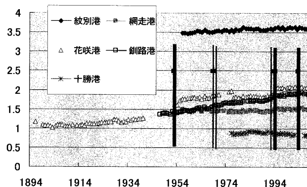
図-4 年平均潮位（東側）
