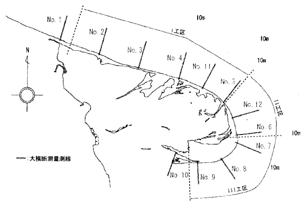
図-6 測量断面位置図
