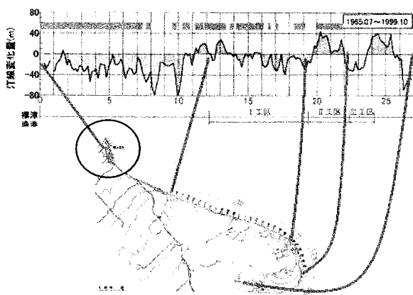
図-8 野付半島の汀線変化図(1965～1999)
