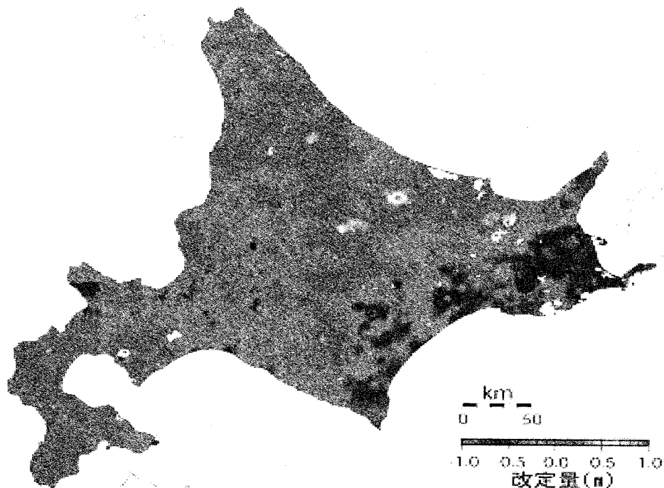
図-1 三角点の標高改定量図
