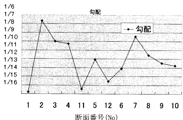
図-7 各断面の勾配値
