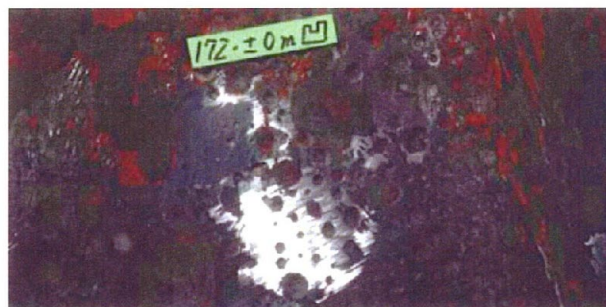
写真-4 鋼矢板の孔食 (L. W. L. 付近)
