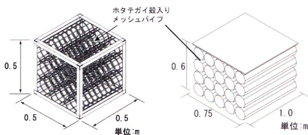
図-3 保護育成ユニット (左: A 型、右: B 型)
