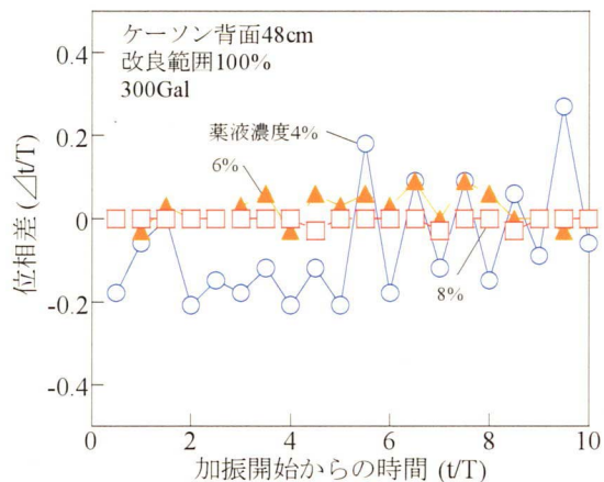
図-5 ケーソン、固化処理および未処理地盤の位相差
