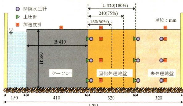
図-1 模型土槽
