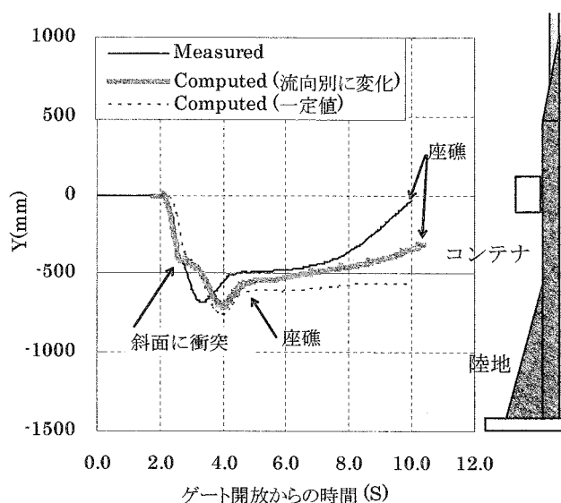
図-10 実験結果と解析結果の漂流軌跡の比較 (設置角 0°, 水位差 0.2m)
