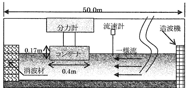
図-3 抗力実験の模式図
