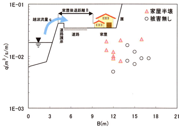
図-2 家屋被害発生時の越波流量
